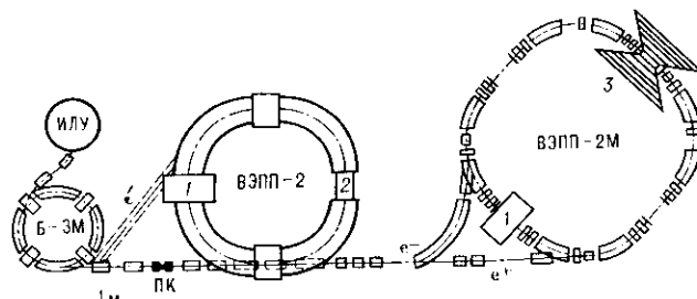
Рис. 1. Схема комплекса установок со встречными электрон-позитронными пучками ВЭП-2М; ИЛУ — импульсный линейный ускоритель электронов, форинджер, энергия 1,5 МэВ, ток в импульсе 30 А ( 3 \cdot 10^{11} частиц); В-3М — синхротрон на энергию 360 МэВ, 3 \cdot 10^{11} частиц за цикл, частота повторения 1 Гц; ПК — позитронный конвертер; ВЭП-2 — промежуточный накопитель на энергию 650 МэВ; 1 — резонаторы ВЧ-системы; 2 — участок регистрации ВЭП-2 во время работы в качестве накопителя со встречными e^+e^- -пучками (пунктиром показан существовавший в то время канал инжекции электронов); ВЭП-2М — действующий накопитель со встречными e^+e^- -пучками; 3 — детектор.
