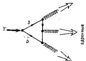
Рис. 12. Распад \Upsilon -частицы в три адронные струи.
