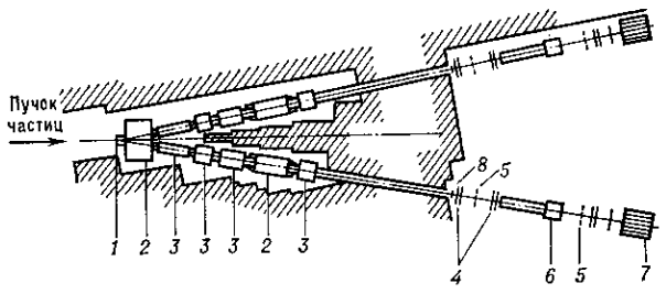
Рис. 2. Схема двухплечевого магнитного спектрометра: 1 — мишень; 2 — магниты; 3 — магнитные линзы; 4 — трековые детекторы; 5, 8 — сцинтилляционные детекторы; 6 — газовые черенковские счётчики; 7 — ливневые спектрометры для идентификации электронов.
