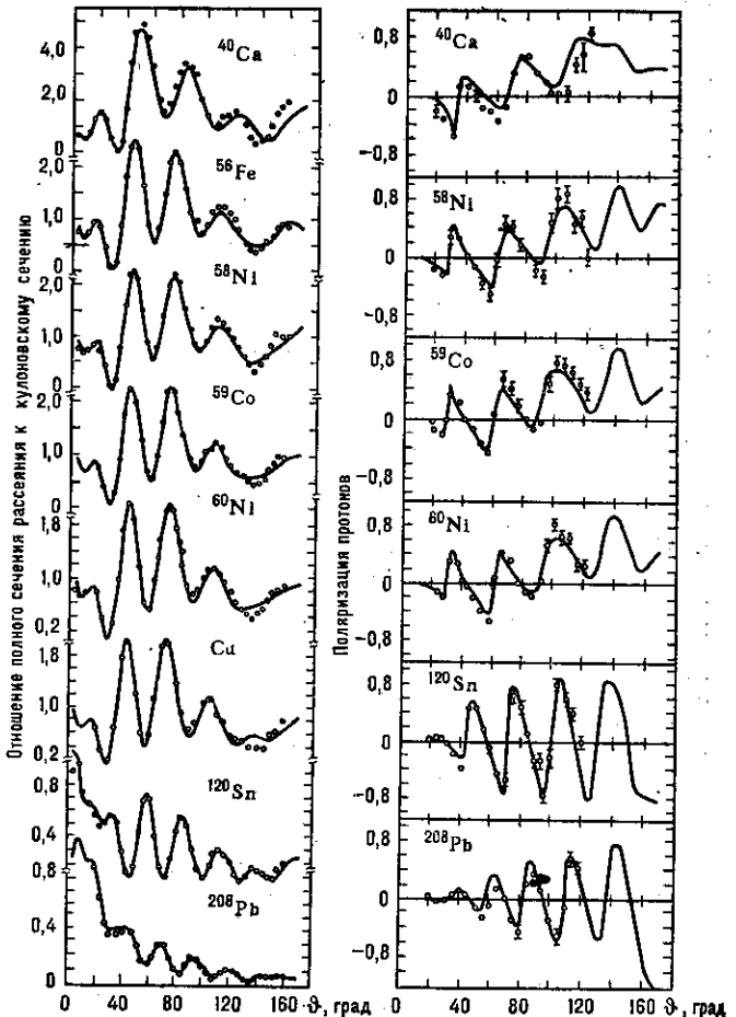
Рис. 1. Дифференциальные сечения рассеяния и поляризации для рассеяния протонов на ряде ядер в зависимости от угла рассеяния \theta в системе центра масс.
