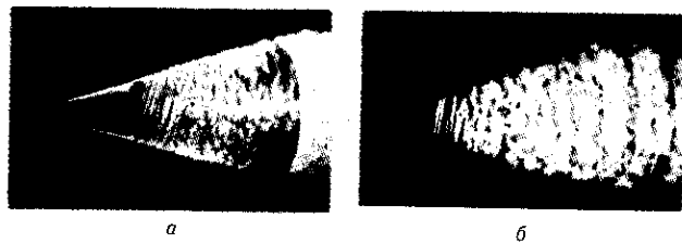
Рис. 8. Развитие турбулентности из спиральных вихрей, формирующихся в пограничном слое при обтекании вращающегося конуса: а) U = 1,7 м/с; n = 670 об/мин; б) U = 1,0 м/с; n = 1200 об/мин. Здесь U — скорость набегающего потока, n — частота вращения (R. Kobayashi, L. Kohama, M. Kurosawa, 1983).
